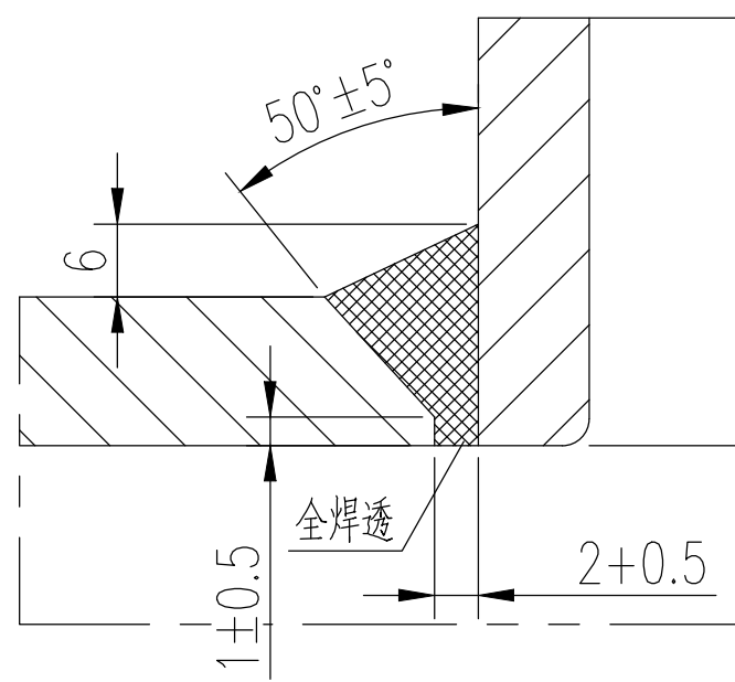
径向接管与壳体焊接详图
