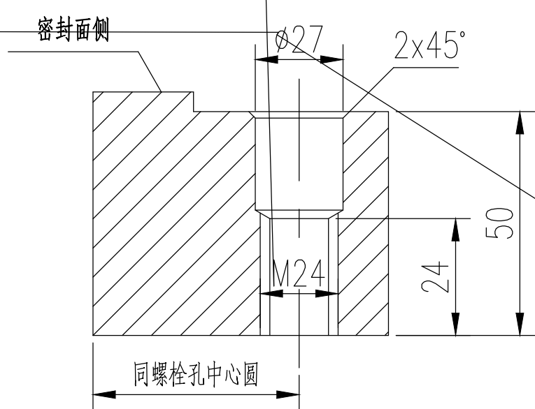
顶丝孔详图
