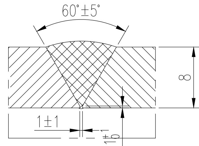
A,B类对接接头详图
