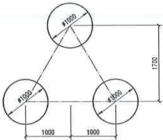
振冲碎石桩位布置示意图
